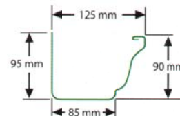
Perfiles de Canalones
